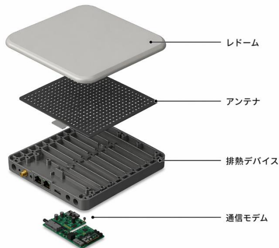
図3 排熱デバイスとNTN向け平面アンテナ、通信モデムを統合した衛星通信ユーザー端末の構成イメージ
