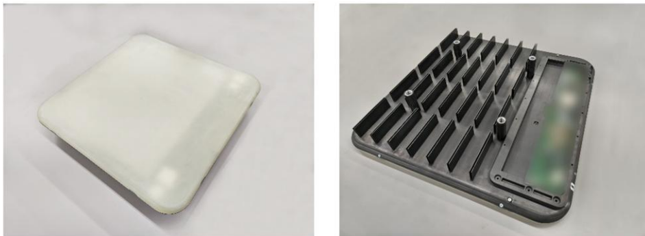
図2 開発したNTN向け平面アンテナ（約45cm四方） 左: 表側外観、右: 裏側外観
